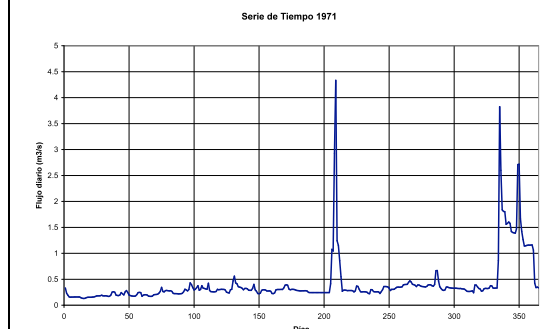
Figura 5. Serie de tiempo flujos promedio diarios. Estación Conchos (Clave 24242)
