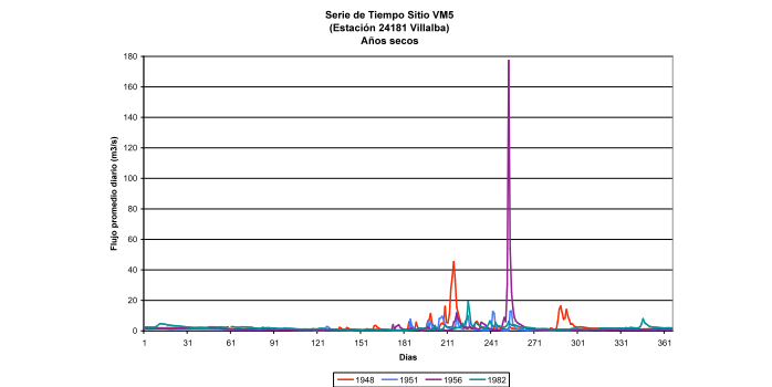
Figura 5: Serie de tiempo flujos promedio diarios. Estación Villalba (Clave 24181)
