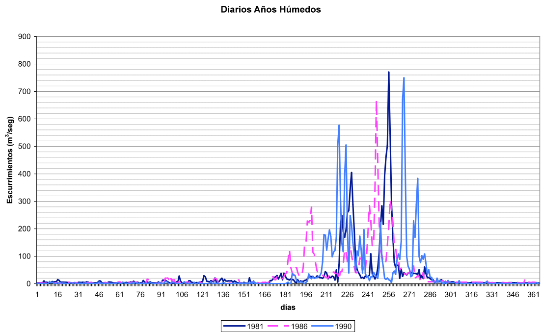
Figura 8. Escurreimientos diarios VM5 San Pedro de Conchos, para tres años húmedos en metros cúbicos por segundo.
