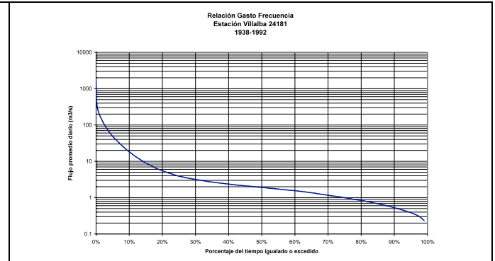
Figura 4: Relación gasto diario-frecuencia. Estación Villalba (Clave 24181) 1938 a 1992.
