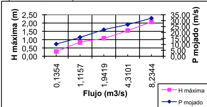
Flujo vs. Profundidad máxima y perímetro mojado
