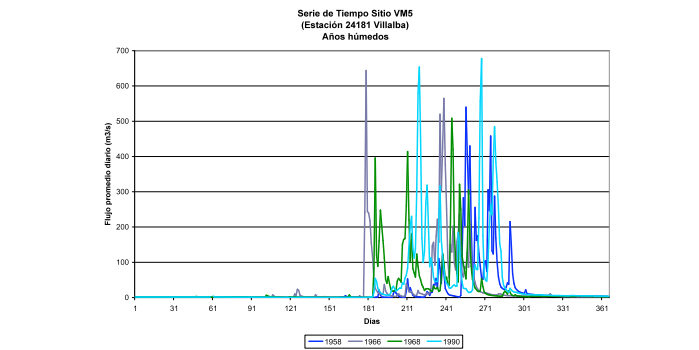
Figura 4: Serie de tiempo flujos promedio diarios. Estación Villalba (Clave 24181)
