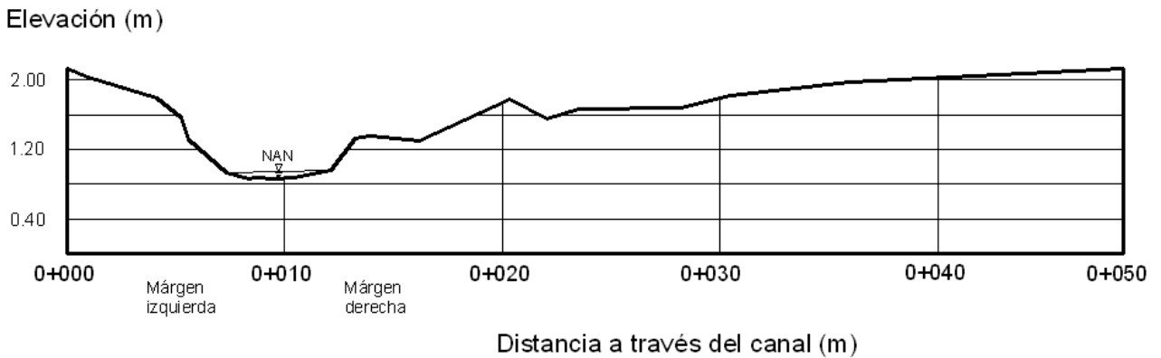
Sección transversal Estación Conchos
