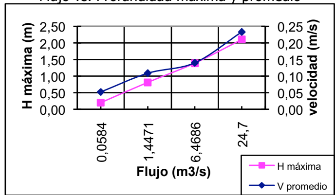
Flujo vs. Profundidad máxima y velocidad
