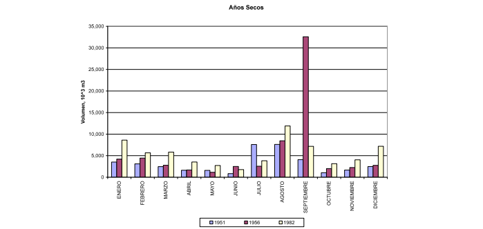
Histograma de volúmenes mensuales para tres años secos. Estación Villalba (Clave 24388)
