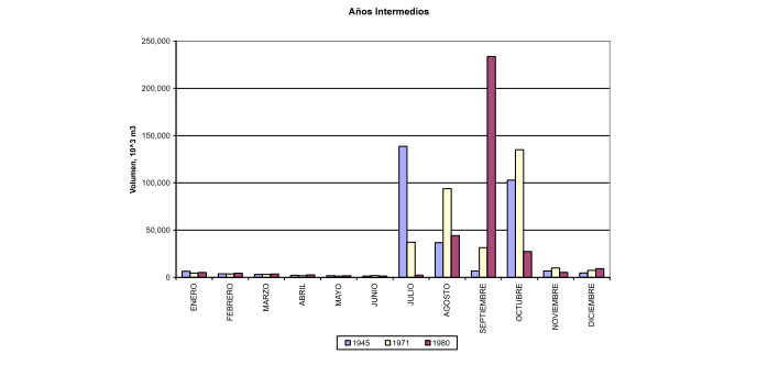
Histograma de volúmenes mensuales para tres años intermedios. Estación Villalba (Clave 24388)
