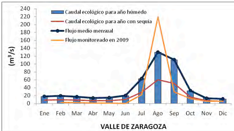
Figura 38. Resultados del monitoreo de flujo en el sitio Valle de Zaragoza
