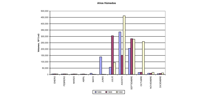
Histograma de volúmenes mensuales para tres años húmedos. Estación Villalba (Clave 24388)
