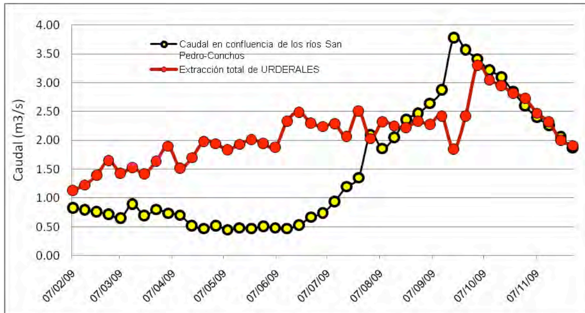
Figura 14. Comparación del flujo entre la extracción de los URDERALES con la descarga del río San Pedro en el río Conchos.
