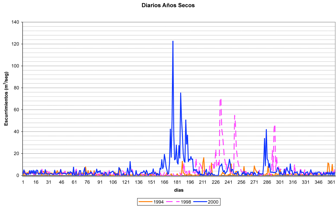
Figura 7. Escurreimientos diarios VM5 San Pedro de Conchos, para tres años secos en metros cúbicos por segundo.
