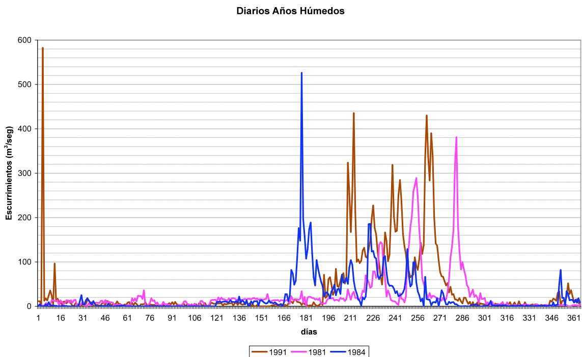
Figura 8. Escurreimientos diarios VMa Valle del Rosario, para tres años húmedos en metros cúbicos por segundo.
