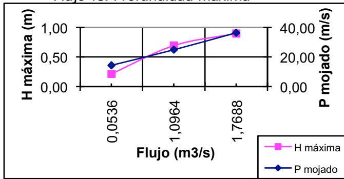
Flujo vs. Profundidad máxima y perímetro mojado
