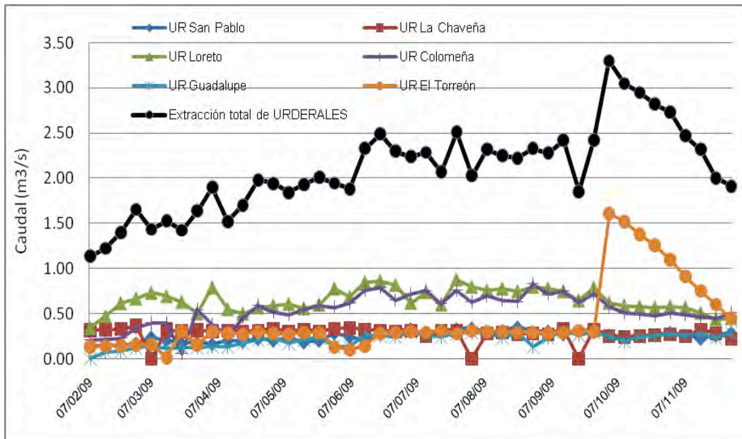
Figura 13. Resultado del monitoreo de la extracción de agua por las URDERALES en el río San Pedro.
