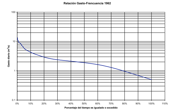
Relación gasto diario-frecuencia para 1962. Estación Conchos (Clave 24242)
