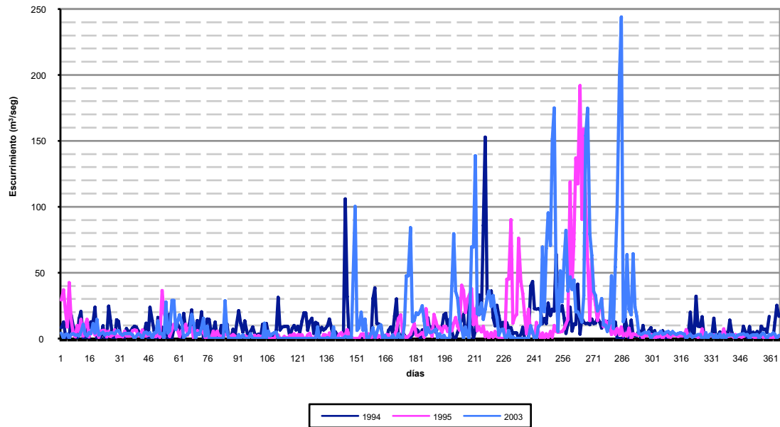
Figura 7. Ecurrimientos diarios VMb Valle de Zaragoza, para tres años secos en metros cúbicos por segundo.
