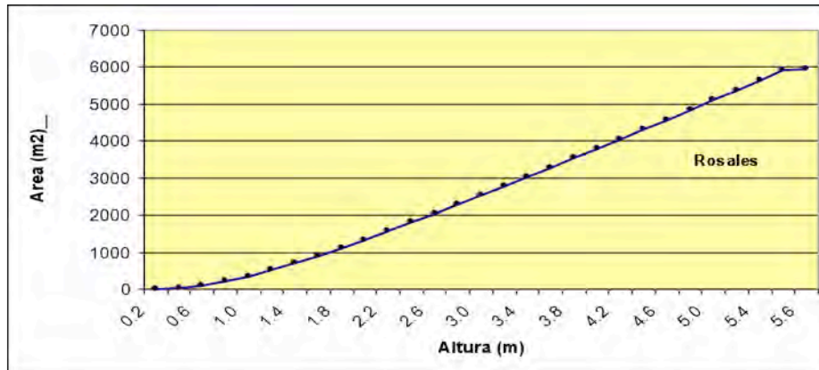
Relación altura-área
