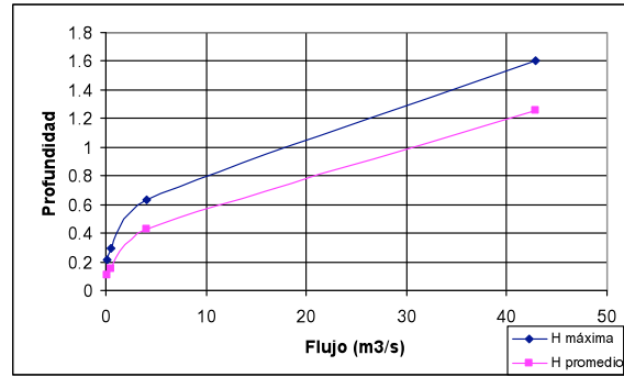
Flujo vs. Profundidad máxima y promedio
