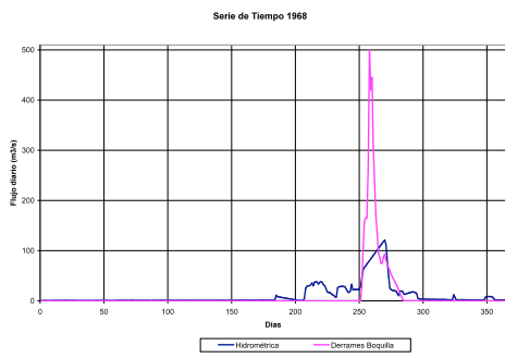
Figura 4. Serie de tiempo flujos promedio diarios. Estación Conchos (Clave 24242) y Derrames de La Boquilla
