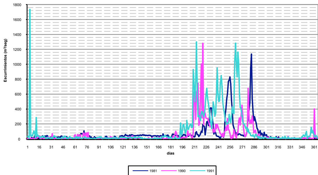
Figura 8. Ecurrimientos diarios VMb Valle de Zaragoza, para tres años húmedos en metros cúbicos por segundo.
