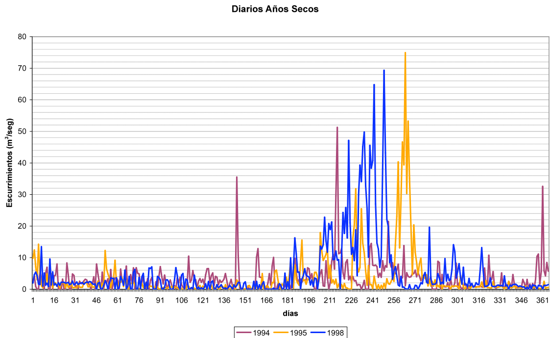
Figura 7. Escurreimientos diarios VMa Valle del Rosario, para tres años secos en metros cúbicos por segundo.
