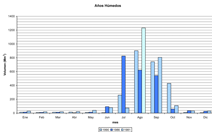
Figura 6. Volúmenes anuales VM5 San Pedro de Conchos, para tres años húmedos en millones de metros cúbicos.
