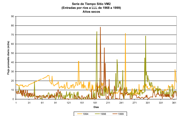
Figura 5: Serie de tiempo flujos promedio diarios. Entradas por ríos a LLL 1968 a 1999.
