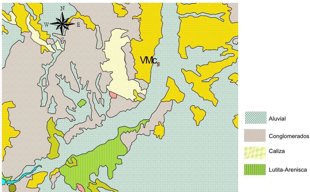
Geología del Sitio VMc Camargo
