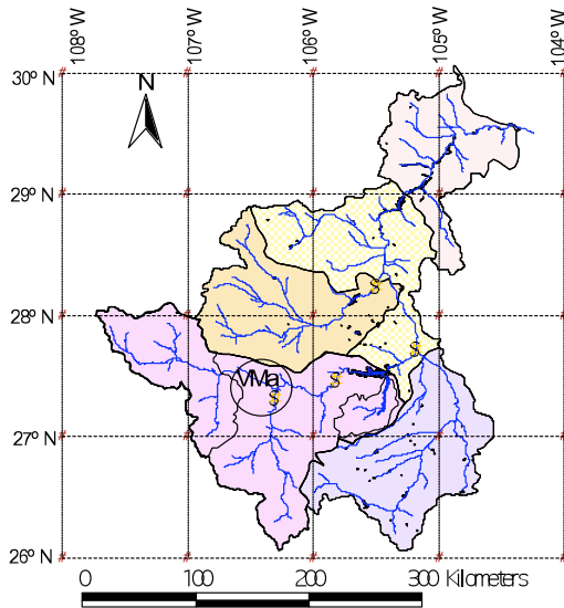
Figura 1. Cuenca río Conchos, localización del sitio de estudio VMa Valle del Rosario.
